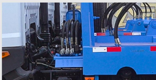
多路阀组 ↑
