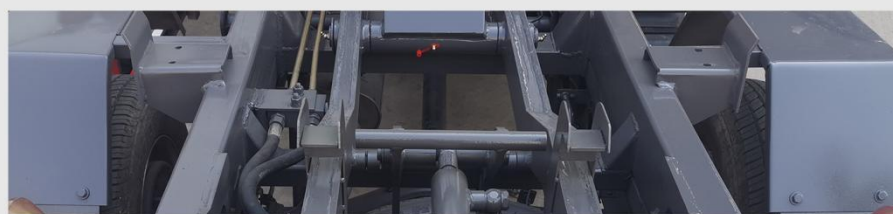
液压横向锁紧 ↑
